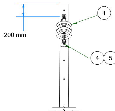
VISTA DE PERFIL ESC: 1 / 35
