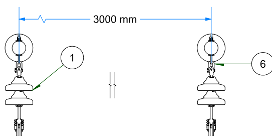
VISTA DE PLANTA ESC: 1 / 35
