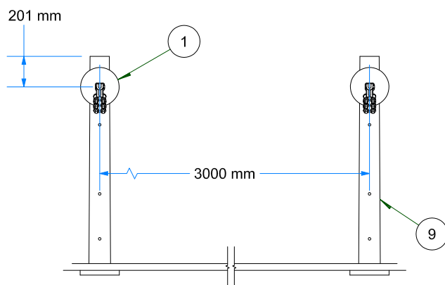
VISTA FRONTAL ESC: 1 / 35
