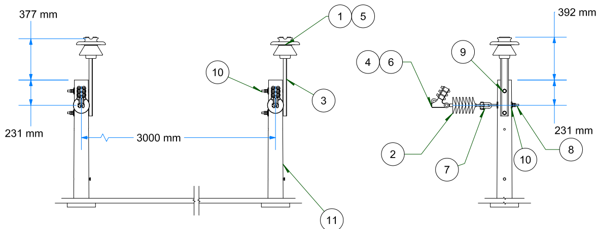
VISTA DE PERFIL ESC: 1 / 35
