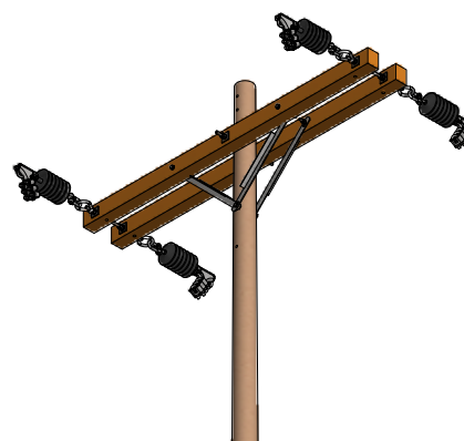
VISTA ISOMETRICA ESC: 1 / 50
