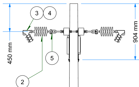
VISTA DE PERFIL ESC: 1 / 35
