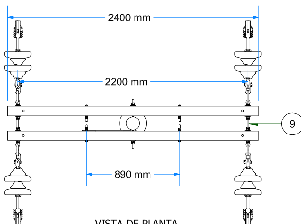
VISTA DE PLANTA ESC: 1 / 35
