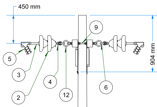
VISTA DE PERFIL ESC: 1 / 35
