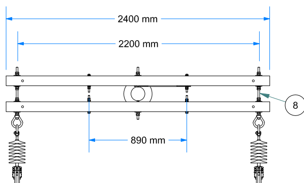
VISTA DE PLANTA ESC: 1 / 35
