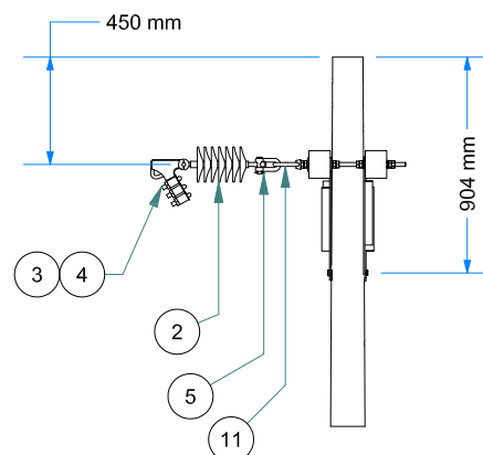
VISTA DE PERFIL ESC: 1 / 35
