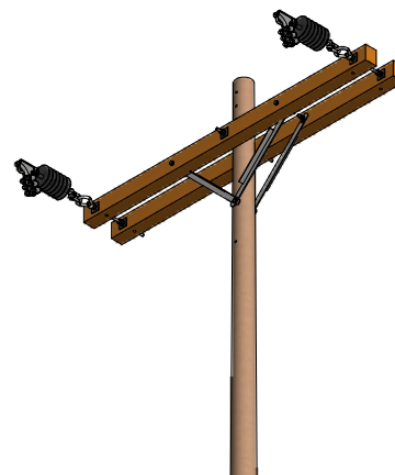
VISTA ISOMETRICA ESC: 1 / 50
