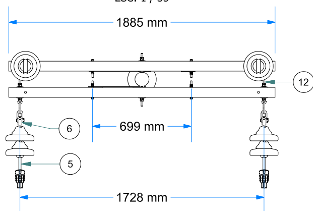
VISTA DE PLANTA ESC: 1 / 35
