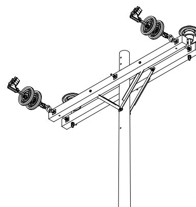
VISTA ISOMETRICA ESC: 1 / 50
