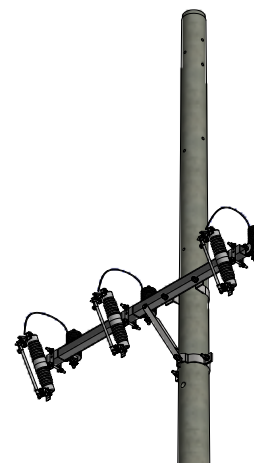
VISTA ISOMETRICA ESC: 1 / 50
