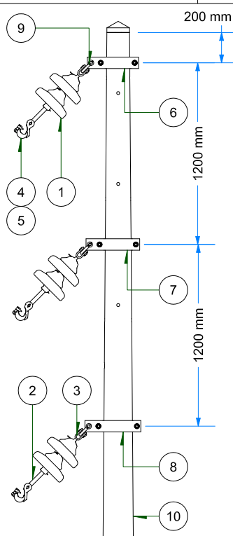
VISTA DE PERFIL ESC: 1 / 35
