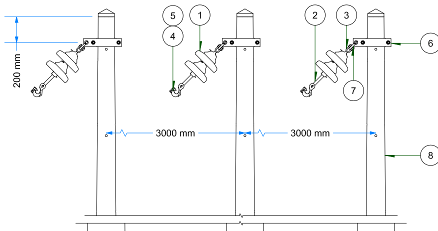
VISTA FRONTAL ESC: 1 / 35
