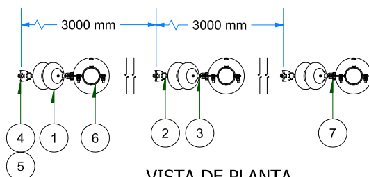
VISTA DE PLANTA ESC: 1 / 50
