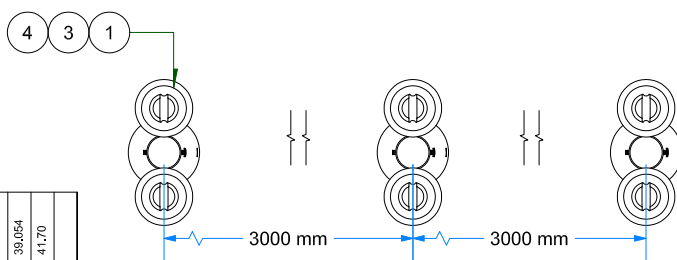
VISTA DE PLANTA ESC: 1 / 35
