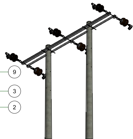
VISTA ISOMETRICA ESC: 1 / 75
