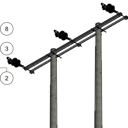
VISTA ISOMETRICA ESC: 1 / 75
