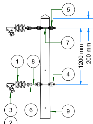
VISTA DE PERFIL ESC: 1 / 50
