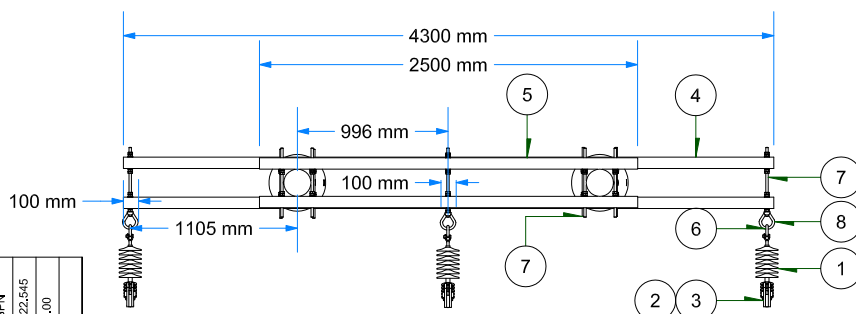
VISTA DE PLANTA ESC: 1 / 50
