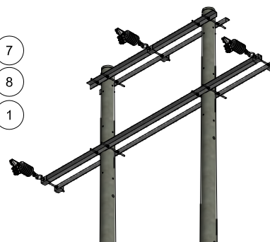
VISTA ISOMETRICA ESC: 1 / 75
