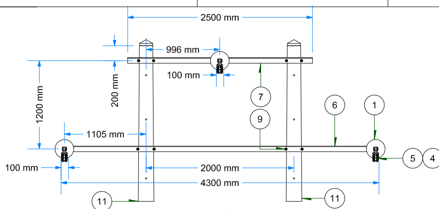
VISTA FRONTAL ESC: 1 / 50
