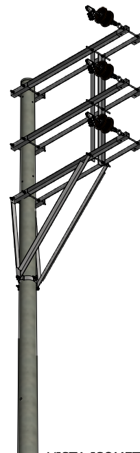
VISTA ISOMETRICA ESC: 1 / 75
