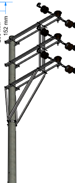
VISTA ISOMETRICA ESC: 1 / 75
