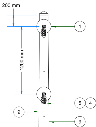
VISTA FRONTAL ESC: 1 / 35
