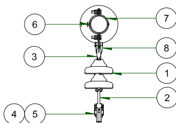
VISTA FRONTAL ESC: 1 / 35
