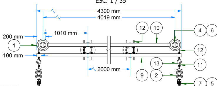
VISTA DE PLANTA ESC: 1 / 50
