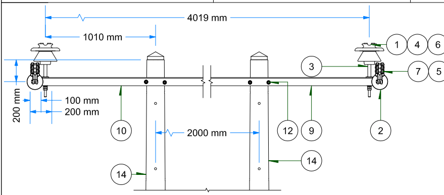
VISTA FRONTAL ESC: 1 / 35
