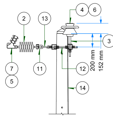
VISTA DE PERFIL ESC: 1 / 35
