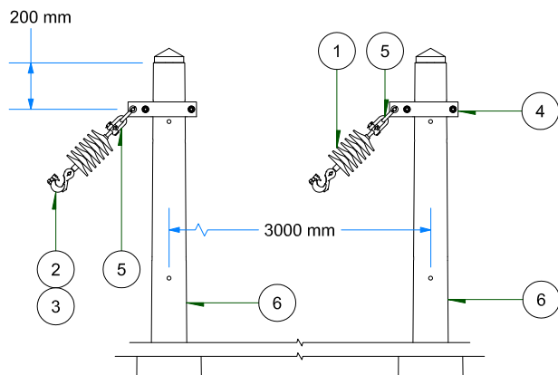
VISTA FRONTAL ESC: 1 / 35
