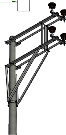
VISTA ISOMETRICA ESC: 1 / 75
