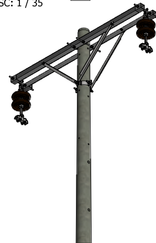
VISTA ISOMETRICA ESC: 1 / 50
