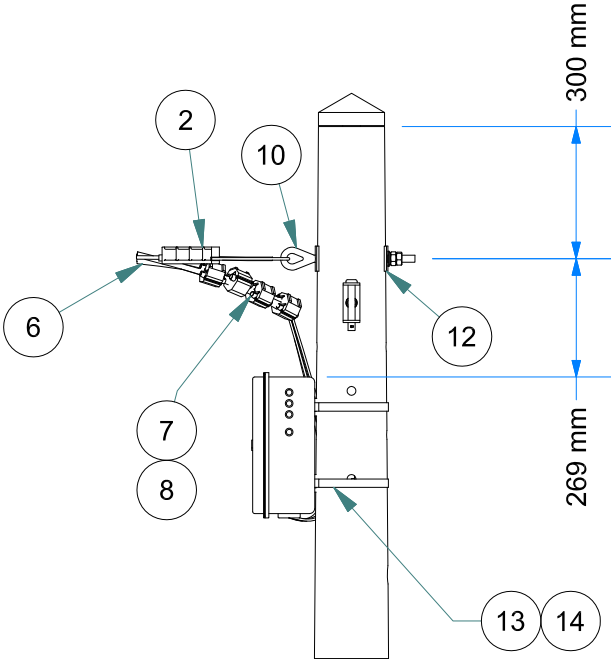
VISTA DE PERFIL ESC: 1 / 25
