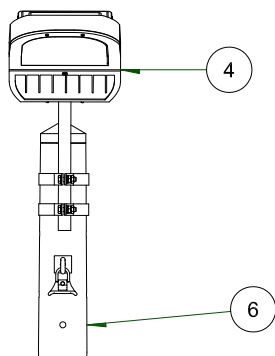
VISTA FRONTAL ESC: 1 / 25
