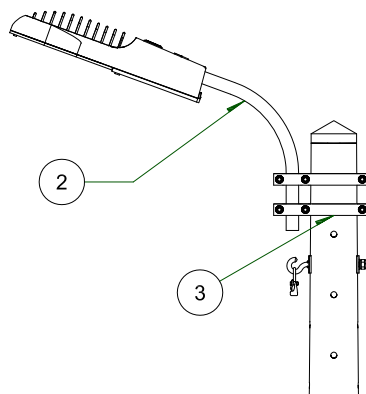
VISTA DE PERFIL ESC: 1 / 25
